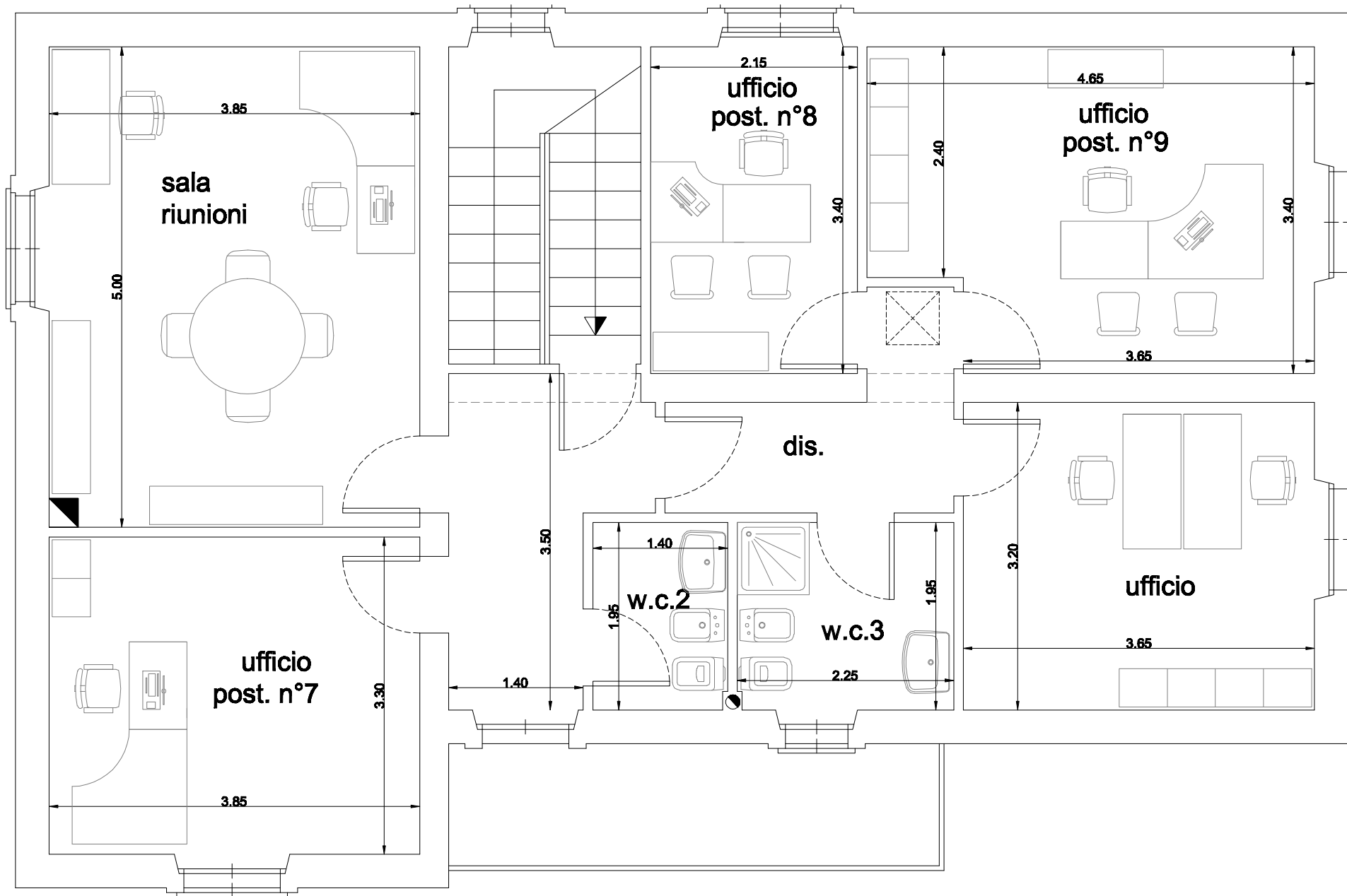
PIANTA UFFICI PIANO PRIMO postazioni n°3
